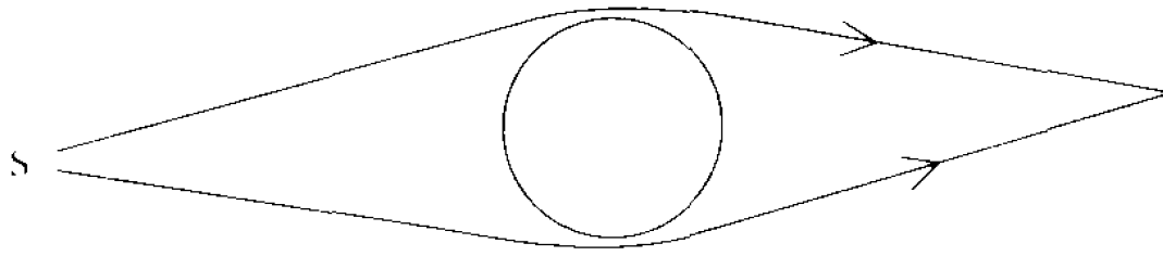
Abbildung 7: Eine Gravitationslinse. Die Schwerkraft des massereichen Körpers (Kreis) lenkt die von der fernen Quelle S kommenden Lichtstrahlen ab. In einem günstigen Fall entstünde dabei ein Brennpunkt. Ein darin befindlicher Beobachter nähme um den Körper herum einen Lichtkreis wahr.
